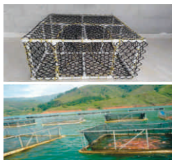
MALLA NASA Color Negro / Verde Producto Ancho Largo Nasa 40 x 40 2 mts 30 mts
